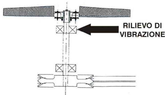
Εικόνα 1-2: Συνιστώμενη θέση για σημεία μέτρησης κραδασμών.
