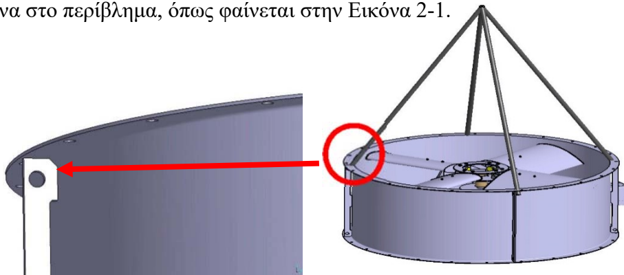
Εικόνα 2-1: Σημεία αγκύρωσης για το χειρισμό του ανεμιστήρα
