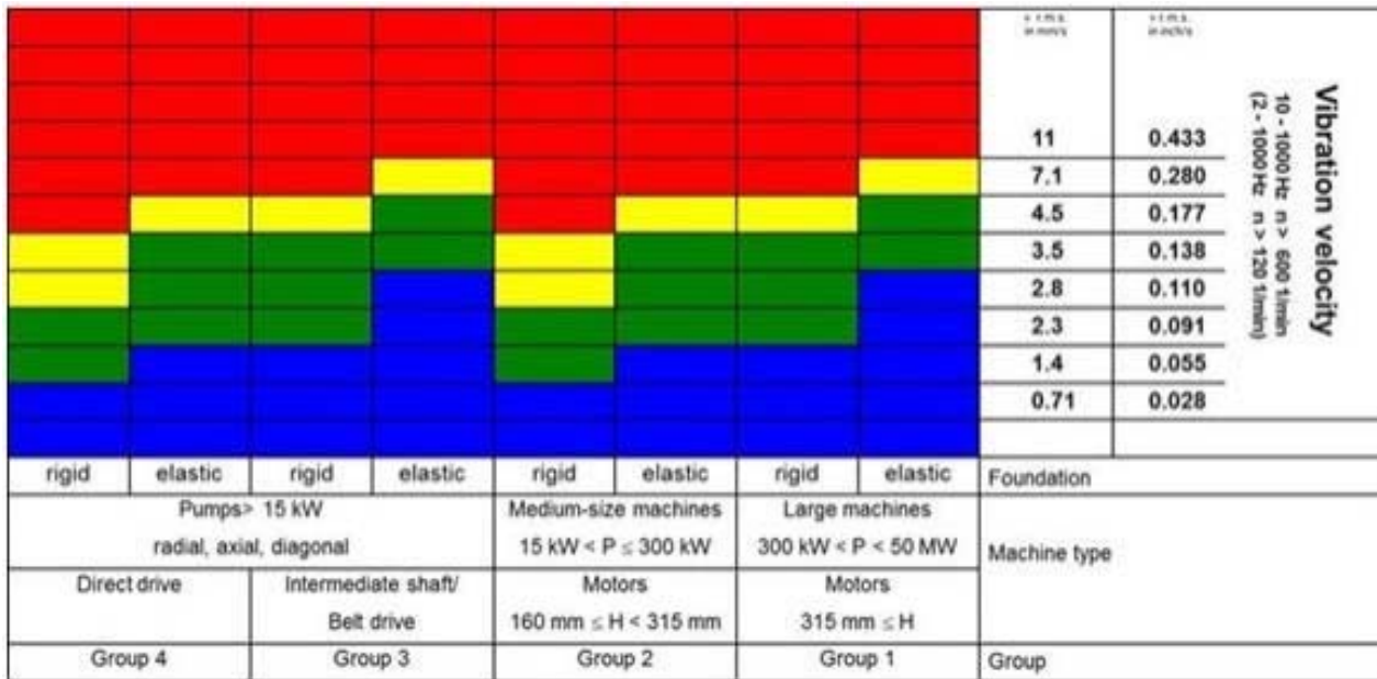
Εικόνα 1-3: Κριτήρια αξιολόγησης κραδασμών κατά ISO 10816.
